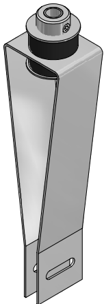
Typ HG 40T / type HG 40T
